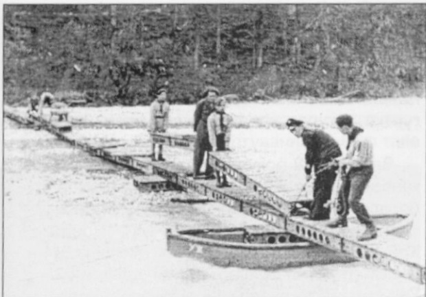
▲ Чорноморці будують міст на Ізарі, 1947
